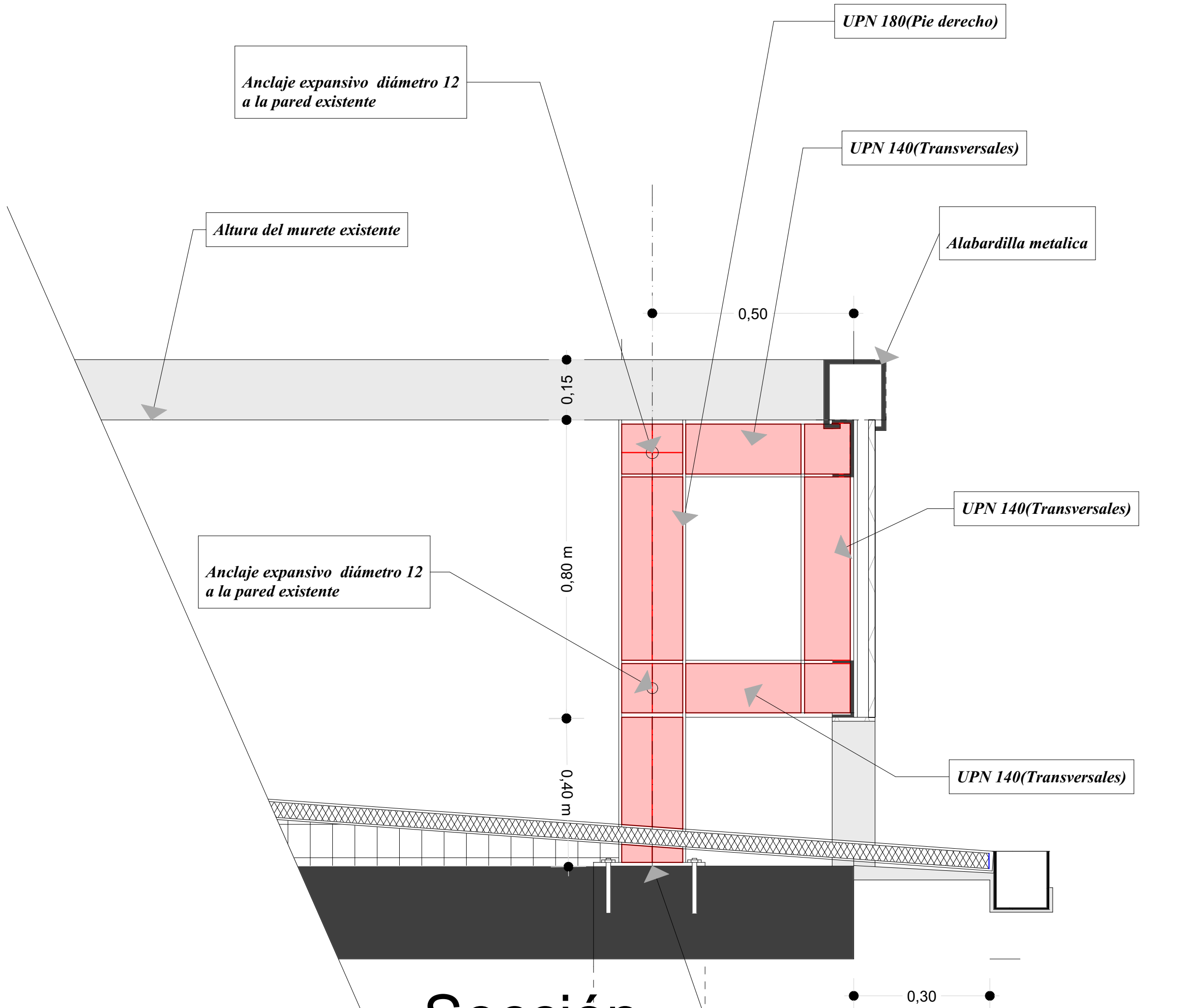
Sección
